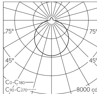
LED 0 K 114 W 13010 lm-h / CIE Flux 44 75 92 90 100 / A42 nach DIN 5040
