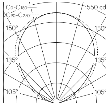
LED 4000 K 12.5 W 1163 lm-h / CIE Flux 0 0 0 100 / E83 nach DIN 5040
