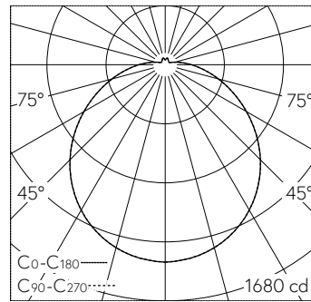
LED 3000 K 48 W 4850 lm-h / CIE Flux 43 72 90 92 100 / A31 nach DIN 5040
