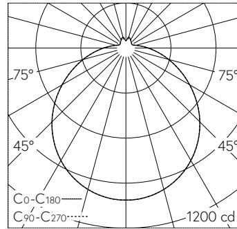
LED 3000 K 48 W 3703 lm-h / CIE Flux 42 71 89 88 100 / B31 nach DIN 5040
