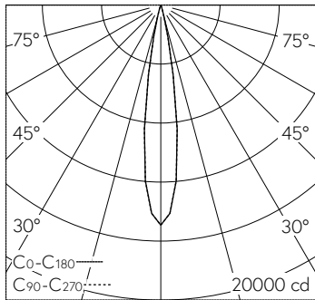
LED 3000 K 20.5 W 2060 lm-h 16.4° / CIE Flux 100 100 100 100 100 / A80 nach DIN...
