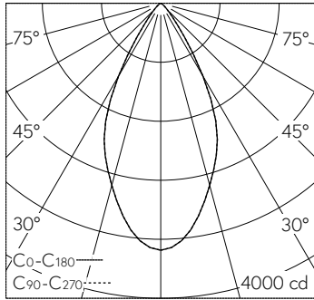
LED 38.6 W 2315 lm-h 52° / CIE Flux 95 100 100 100 / A80 nach DIN 5040
