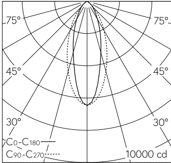
LED 4000 K 39 W 3858 lm-h 30°/44° B10019 / CIE Flux 87 99 100 100 100 / A80 nach DI...
