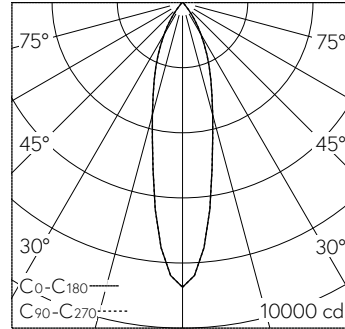
LED 4000 K 39 W 3007 lm-h 24° B71112 / CIE Flux 96 99 100 100 100 / A80 nach DI...
