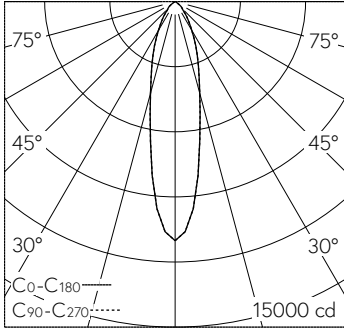
LED 4000 K 39 W 4289 lm-h 24° / CIE Flux 89 99 100 100 100 / A80 nach DIN 5040
