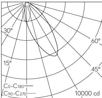
LED 4000 K 39 W 3316 lm-h 30° B10019 / CIE Flux 73 96 100 100 100 / A60 nach DI...
