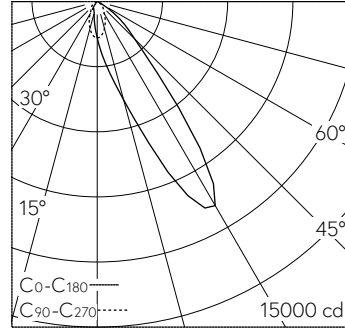
LED 4000 K 39 W 3655 lm-h 30° / CIE Flux 79 98 100 100 100 / A70 nach DIN 5040
