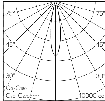
LED 4000 K 13.5 W 875 lm-h 20° B71215 / CIE Flux 98 100 100 100 100 / A80 nach DIN 5040
