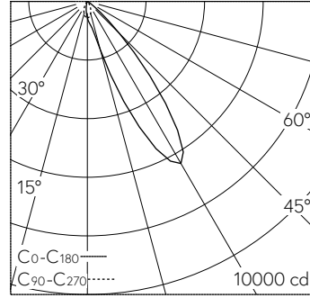
LED 3000 K 13.5 W 1564 lm-h 22° / CIE Flux 95 100 100 100 100 / A80 nach DIN 5040
