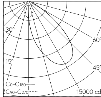
LED 3000 K 69 W 7530 lm-h / CIE Flux 67 96 100 100 100 / A60 nach DIN 5040
