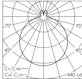
LED 3000 K 13.3 W 1236 lm-h / CIE Flux 45 76 93 86 100 / B43 nach DIN 5040
