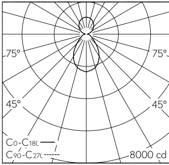
LED 3000 K 68 W 7112 lm-h / CIE Flux 61 84 94 60 100 / B53 nach DIN 5040
