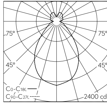
LED 3000 K 68 W 7112 lm-h / CIE Flux 61 83 94 73 100 / B52 nach DIN 5040
