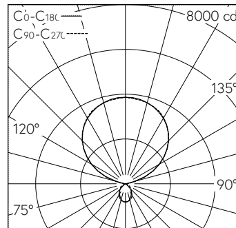
LED 4000 K 82 W 12355 lm-h / CIE Flux 66 92 98 11 100 / D63 nach DIN 5040
