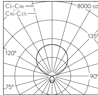
LED 4000 K 82 W 10815 lm-h / CIE Flux 66 92 98 11 100 / D63 nach DIN 5040
