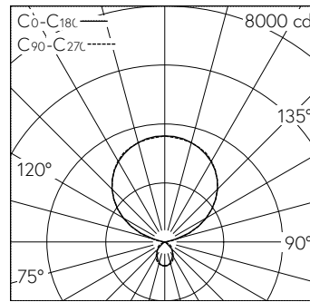
LED 2700 – 6500 K 83 W 11595 lm-h / CIE Flux 66 92 98 12 100 / D63 nach DIN 5040
