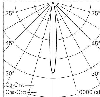
LED 3000 K 9,3 W 535 lm-h 11.0° / CIE Flux 99 100 100 100 / A80 nach DIN 5040
