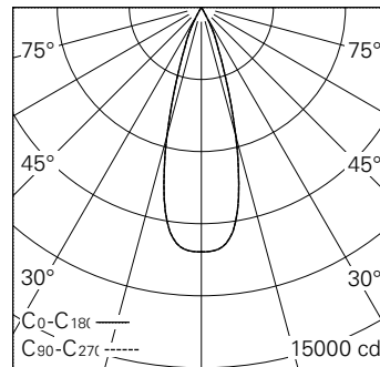
LED 3000 K 42 W 3022 lm-h 32° / CIE Flux 100 100 100 100 100 / A80 nach DIN 5040
