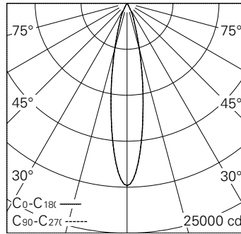
LED 4000 K 36 W 3561 lm-h 20° / CIE Flux 98 100 100 100 100 / A80 nach DIN 5040
