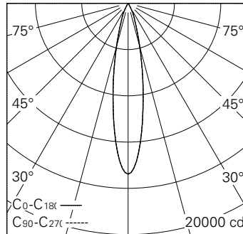
LED 2700 K 36 W 2652 lm-h 20° / CIE Flux 98 100 100 100 100 / A80 nach DIN 5040
