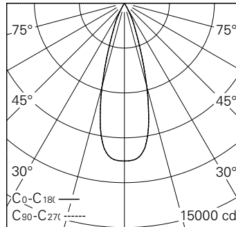
LED 4000 K 27 W 3134 lm-h 32° / CIE Flux 100 100 100 100 100 / A80 nach DIN 5040
