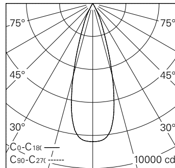
LED 3000 K 27 W 2488 lm-h 32° / CIE Flux 100 100 100 100 100 / A80 nach DIN 5040
