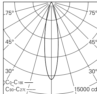
LED 4000 K 20 W 2264 lm-h 20° / CIE Flux 98 100 100 100 100 / A80 nach DIN 5040
