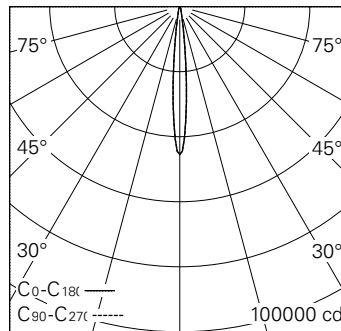
LED 4000 K 20 W 2483 lm-h 10.2° / CIE Flux 100 100 100 100 100 / A80 nach DIN 5...
