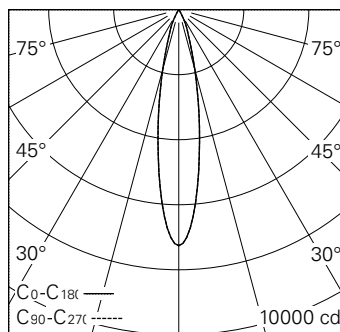
LED 3000 K 14 W 1303 lm-h 20° / CIE Flux 98 100 100 100 100 / A80 nach DIN 5040
