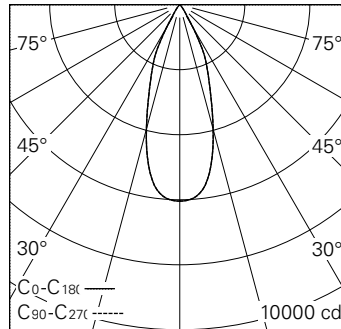
LED 2700 K 27 W 2695 lm-h 38° / CIE Flux 98 100 100 100 100 / A80 nach DIN 5040
