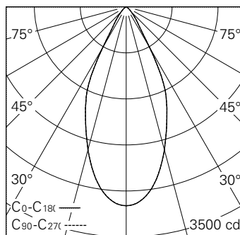
LED 2700 K 20 W 1860 lm-h 48° / CIE Flux 94 99 100 100 100 / A80 nach DIN 5040
