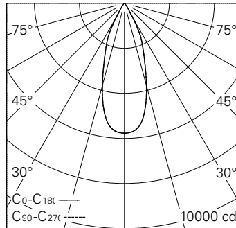
LED 4000 K 20 W 2572 lm-h 38° / CIE Flux 98 100 100 100 100 / A80 nach DIN 5040
