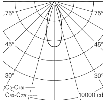
LED 3000 K 20 W 2048 lm-h 38° / CIE Flux 98 100 100 100 100 / A80 nach DIN 5040
