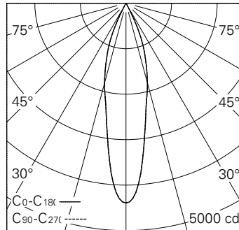
LED 3000 K 14 W 1077 lm-h 24° / CIE Flux 100 100 100 100 100 / A80 nach DIN 5040
