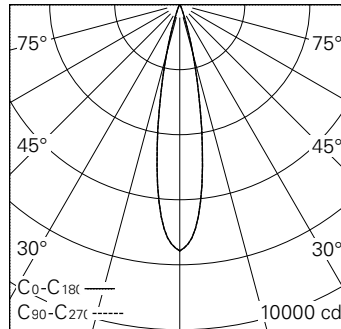
LED 4000 K 11 W 1088 lm-h 20° / CIE Flux 99 100 100 100 100 / A80 nach DIN 5040
