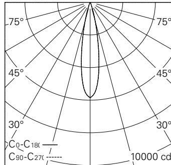
LED 2700 K 11 W 840 lm-h 20° / CIE Flux 99 100 100 100 100 / A80 nach DIN 5040
