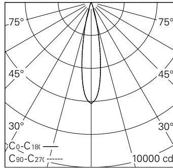
LED 3000 K 11 W 880 lm-h 20° / CIE Flux 99 100 100 100 100 / A80 nach DIN 5040
