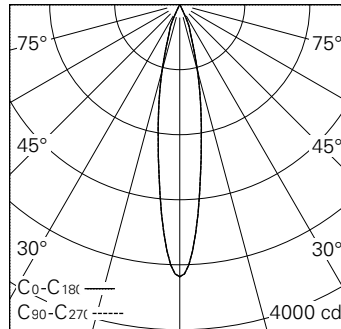
LED 2700 K 11 W 522 lm-h 18.2° / CIE Flux 100 100 100 100 100 / A80 nach DIN 5040
