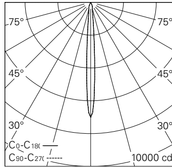
LED 4000 K 4,6 W 392 lm-h 8.0° / CIE Flux 100 100 100 100 100 / A80 nach DIN 5040
