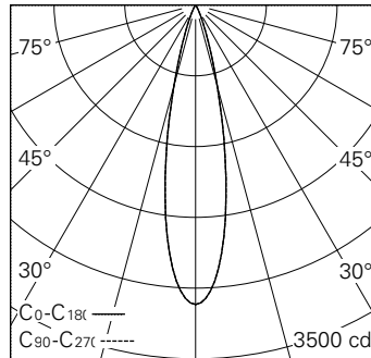
LED 2700 K 11 W 528 lm-h 22° / CIE Flux 99 100 100 100 100 / A80 nach DIN 5040
