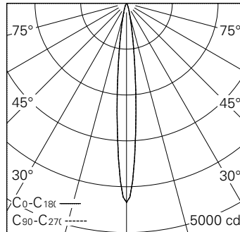
LED 2700 K 4,6 W 310 lm-h 11.0° / CIE Flux 99 100 100 100 / A80 nach DIN 5040
