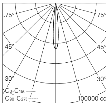
LED 2700 K 36 W 2363 lm-h 11.6° / CIE Flux 96 100 100 100 100 / A80 selon DIN 5...
