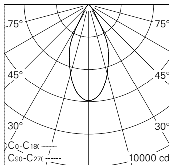
LED 4000 K 31 W 3649 lm-h 48° / CIE Flux 94 99 100 100 100 / A80 selon DIN 5040
