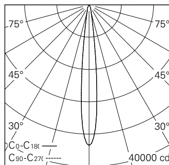
LED 2700 K 27 W 2597 lm-h 12.0° / CIE Flux 100 100 100 100 100 / A80 selon DIN ...
