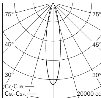
LED 2700 K 42 W 3062 lm-h 20° / CIE Flux 98 100 100 100 100 / A80 selon DIN 5040
