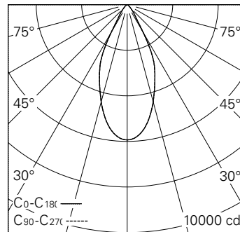
LED 4000 K 31 W 3649 lm-h 48° / CIE Flux 94 99 100 100 100 / A80 selon DIN 5040
