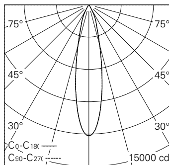
LED 2700 K 31 W 2761 lm-h 22° / CIE Flux 98 100 100 100 100 / A80 selon DIN 5040
