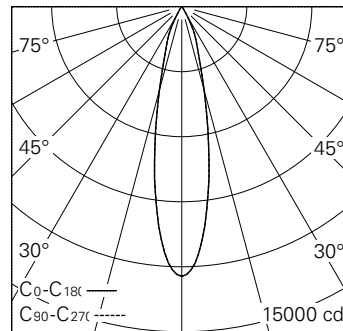
LED 3000 K 31 W 2822 lm-h 22° / CIE Flux 98 100 100 100 100 / A80 selon DIN 5040
