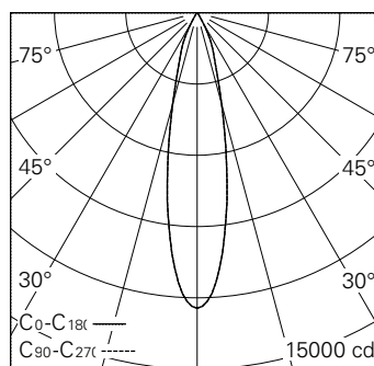
LED 3000 K 31 W 2822 lm-h 22° / CIE Flux 98 100 100 100 100 / A80 selon DIN 5040
