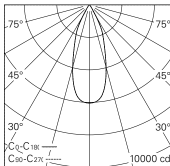
LED 2700 K 27 W 2695 lm-h 38° / CIE Flux 98 100 100 100 100 / A80 selon DIN 5040
