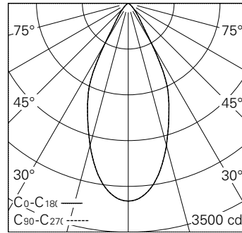
LED 2700 K 20 W 1860 lm-h 48° / CIE Flux 94 99 100 100 100 / A80 selon DIN 5040
