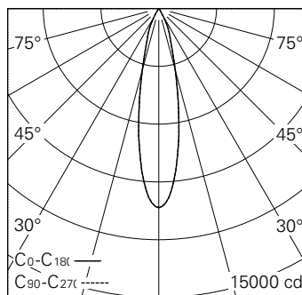
LED 4000 K 20 W 2345 lm-h 22° / CIE Flux 98 100 100 100 100 / A80 selon DIN 5040
