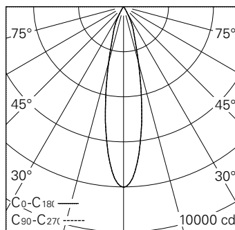
LED 2700 K 20 W 1819 lm-h 22° / CIE Flux 98 100 100 100 100 / A80 selon DIN 5040
