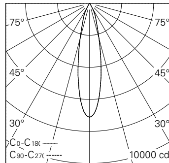
LED 3000 K 20 W 1614 lm-h 22° / CIE Flux 98 100 100 100 100 / A80 selon DIN 5040
